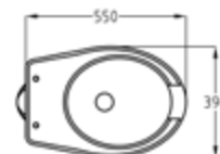
A. Salida suelo
