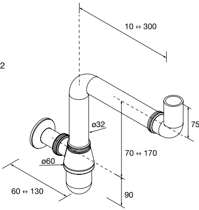
SIFON CONEX
