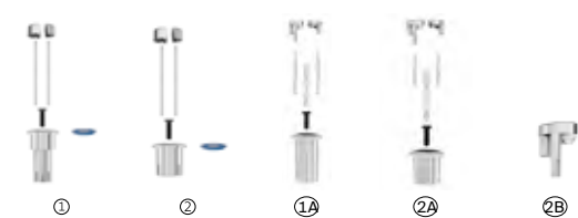
Conjunto doble pulsador 6/3 litros (tapa Ø40)
